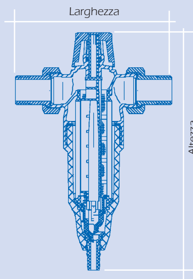
Misure d'ingombro Eurodiago batteriostatico
