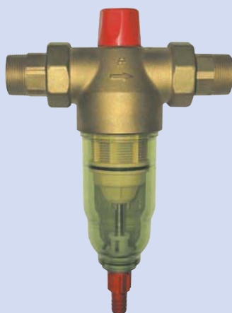
Eurodiago batteriostatico 1 1/2" - 2"
